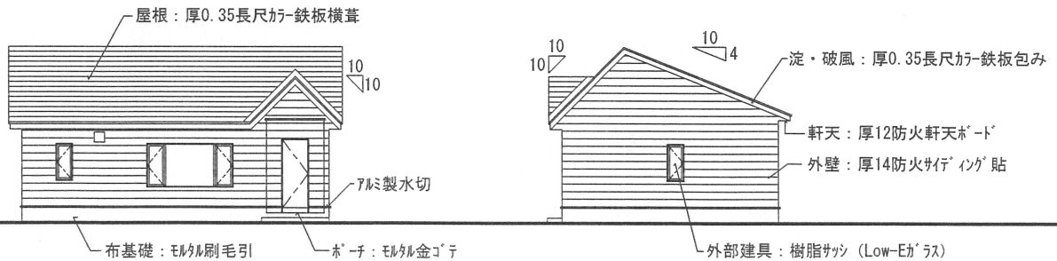
立面図 S=1/200
